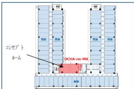
図3 2-7階平面図
